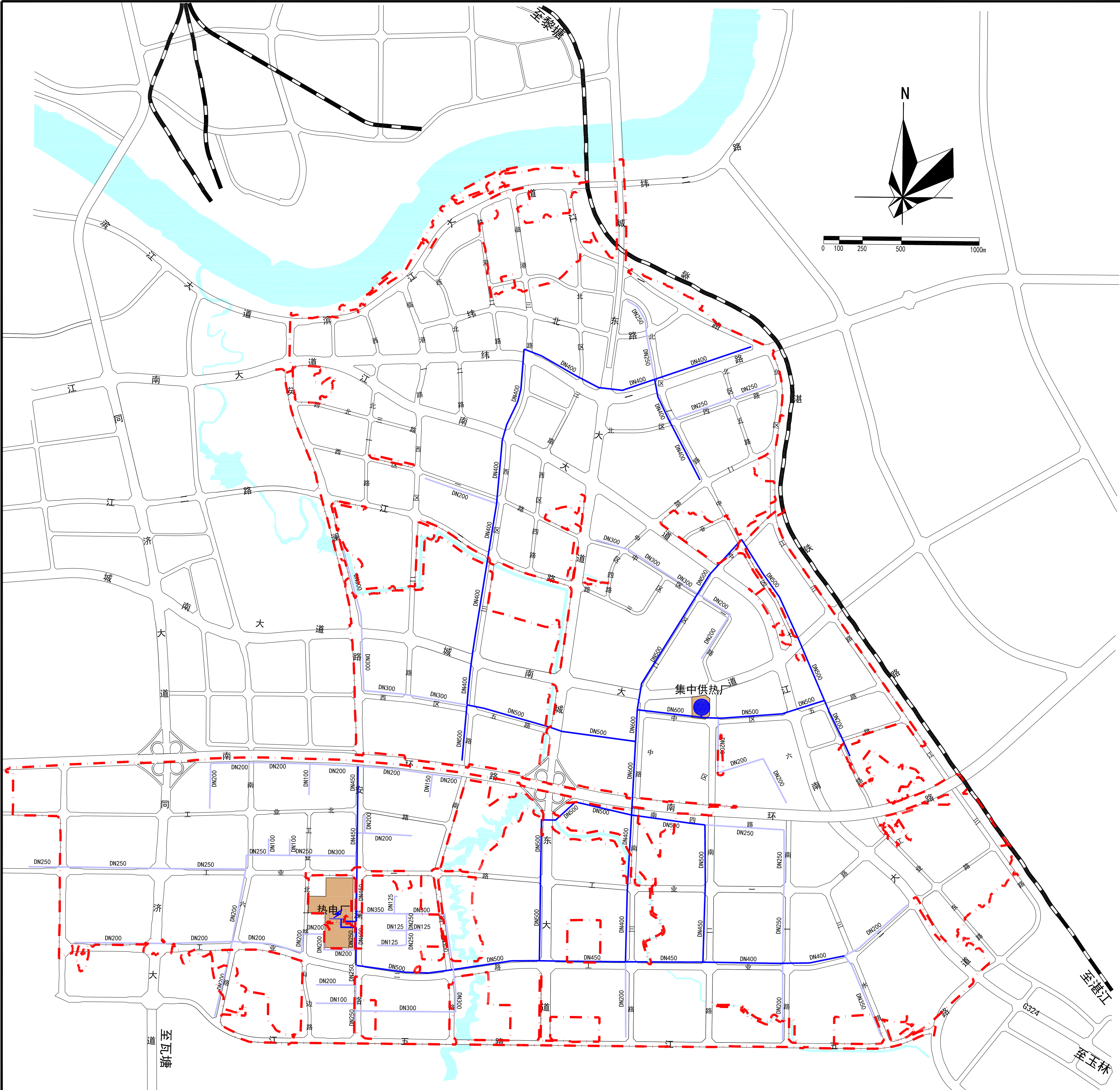
广西贵港江南工业园区控制性详细规划增加供热工程规划方案-供热工程规划图（调整后）
