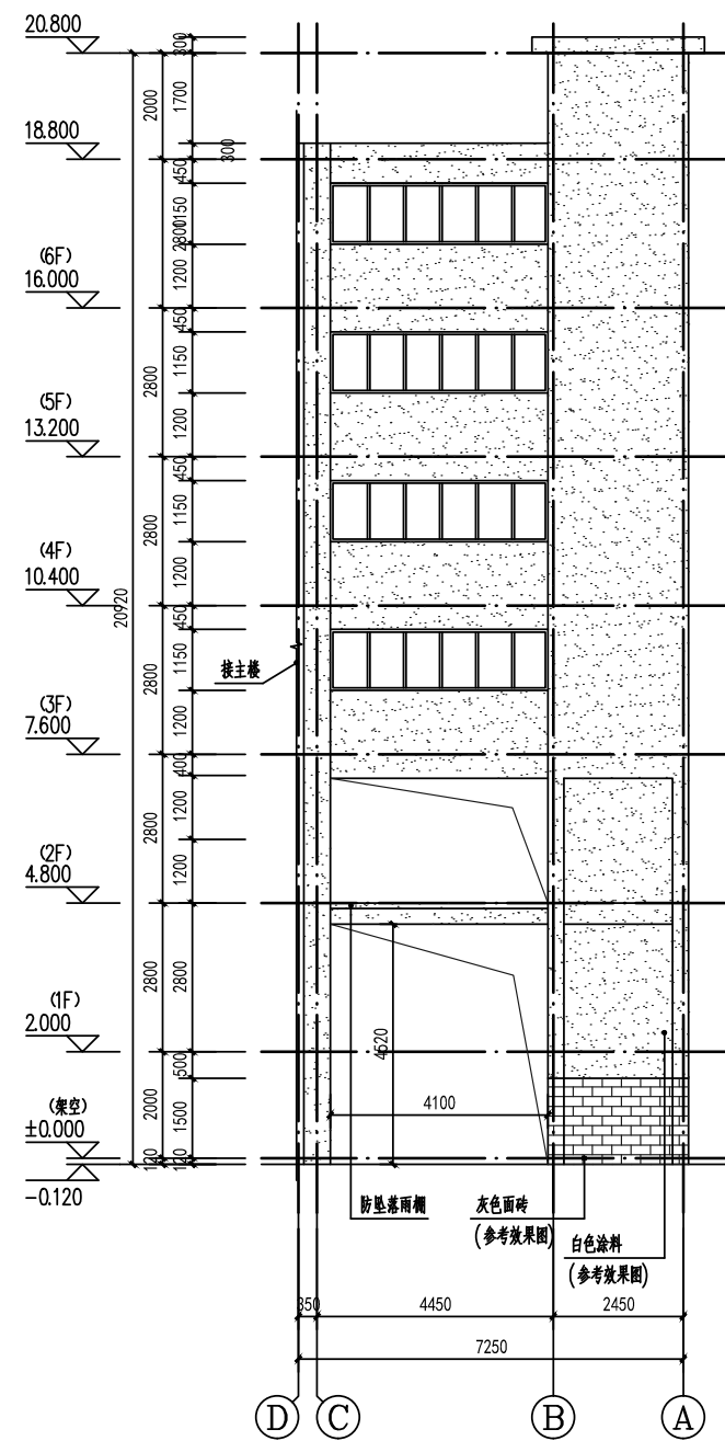
④~①轴立面图 1:100
