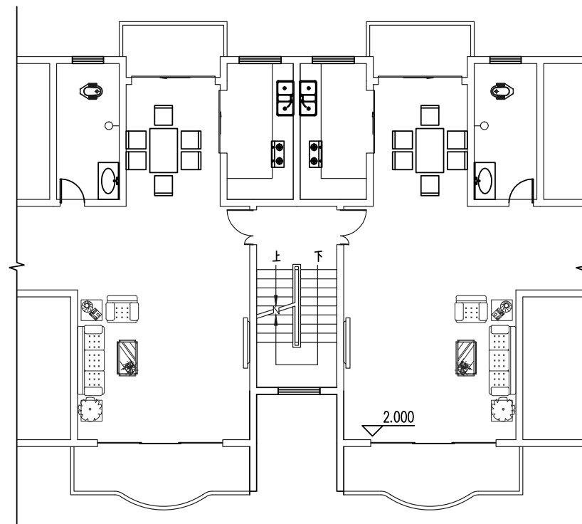
1-2层原始平面图 1:100
