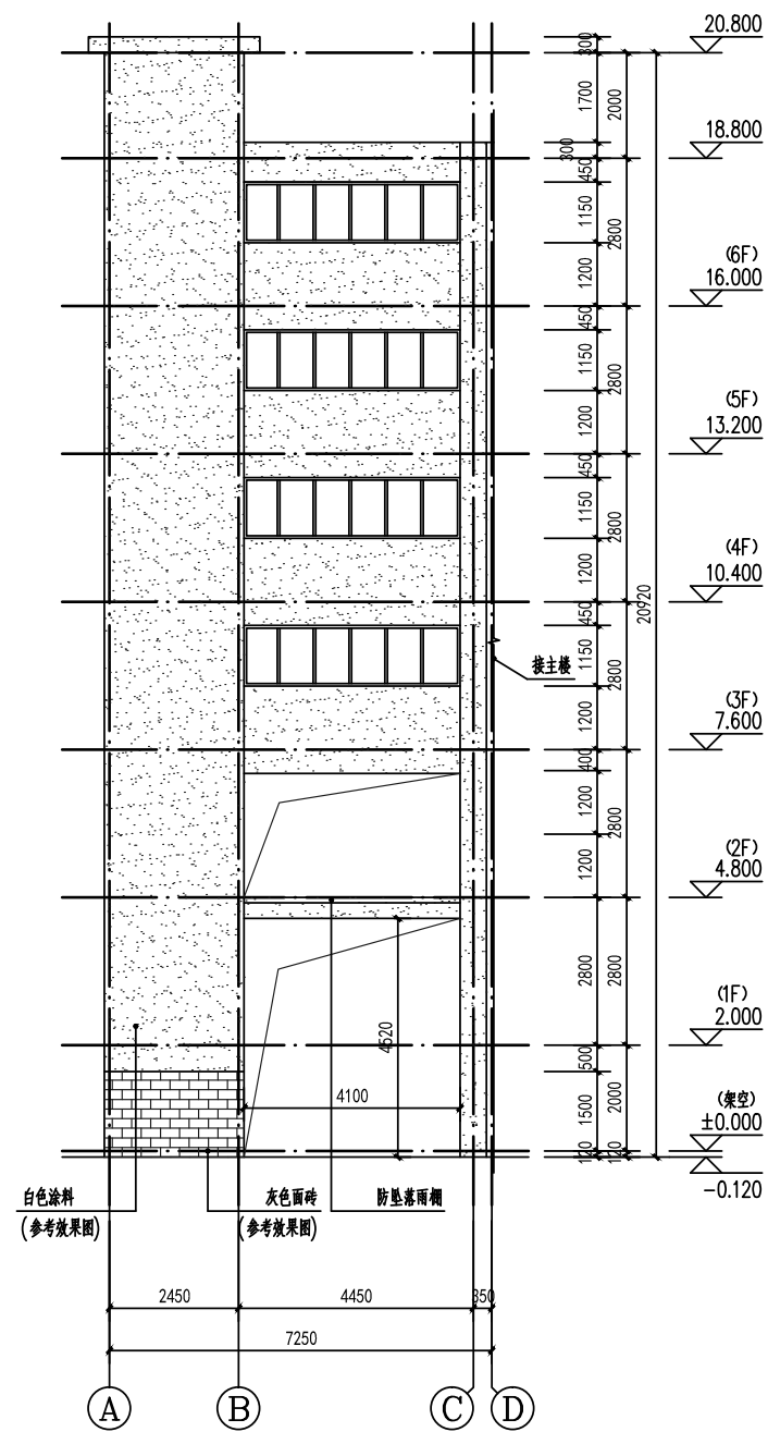
①~④轴立面图 1:100
