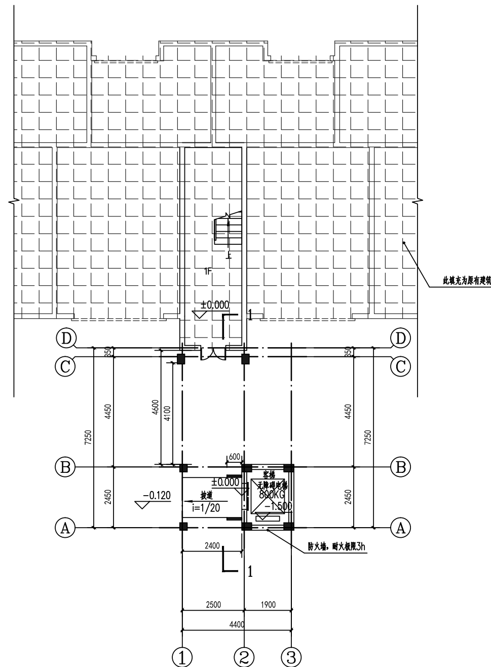
加装电梯后架空层平面图 1:100
