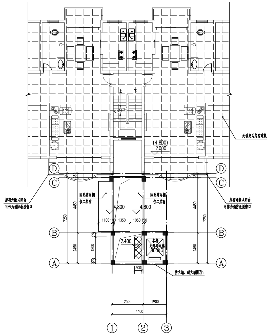
加装电梯后1-2层平面图 1:100
