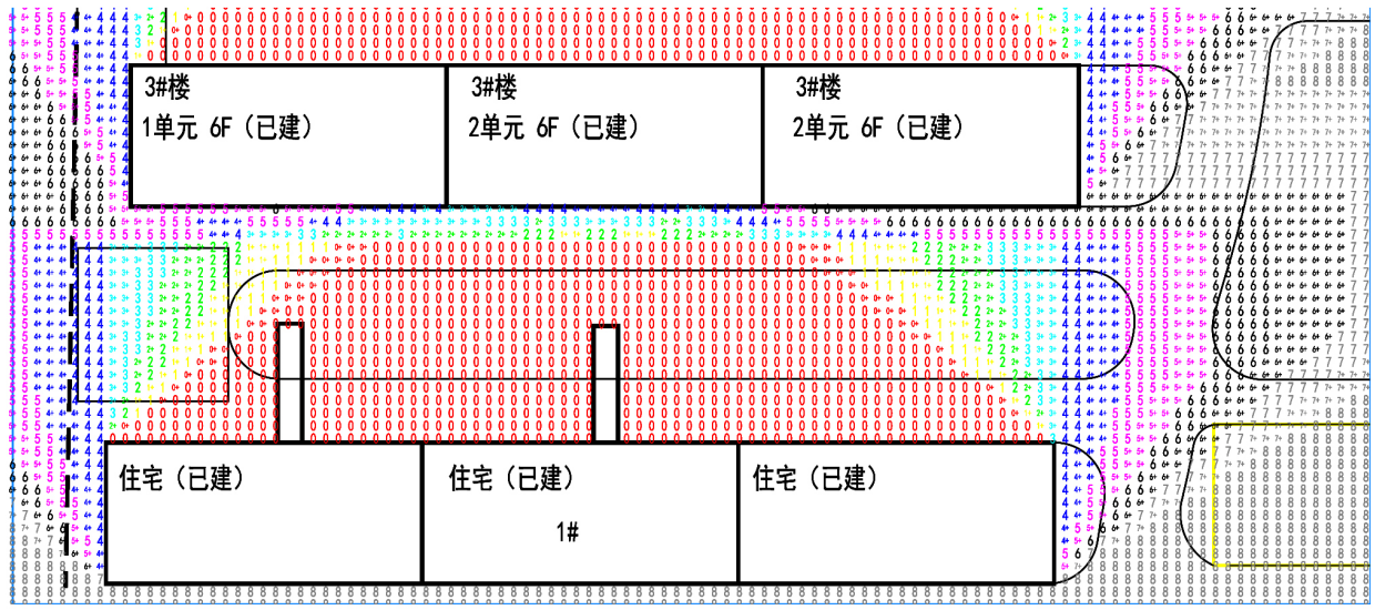
电梯加建前日照分析图
