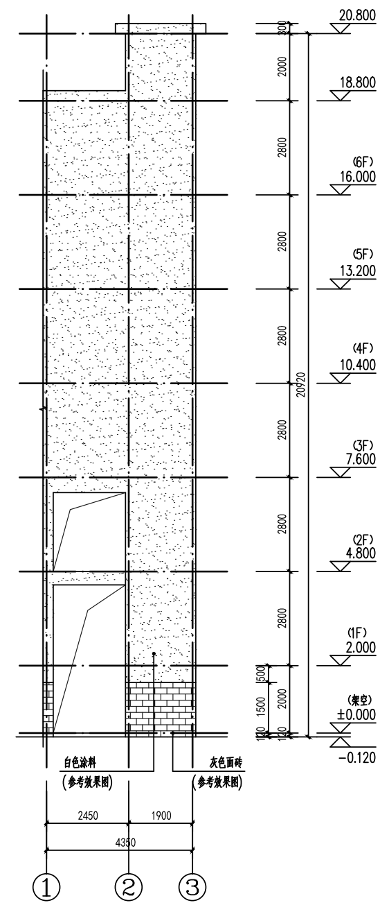
①~③轴立面图 1:100
