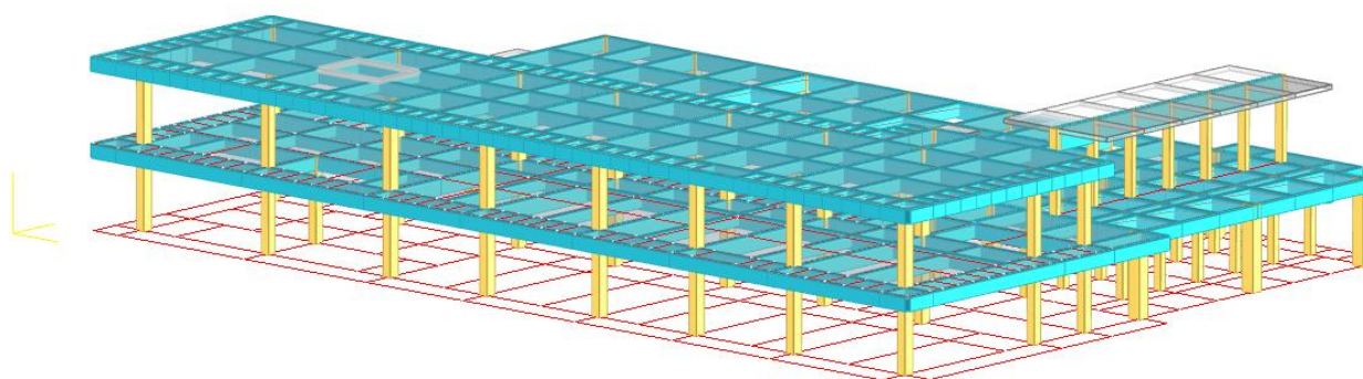
图7.1 结构模型简图
