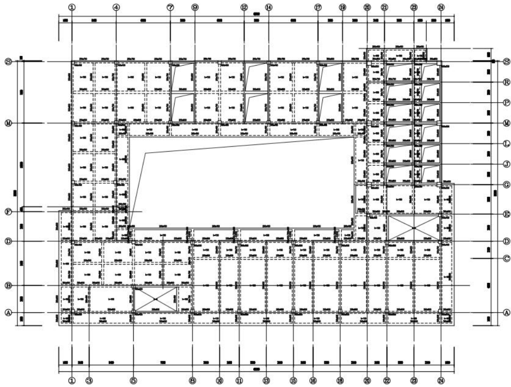
一层结构平面图
