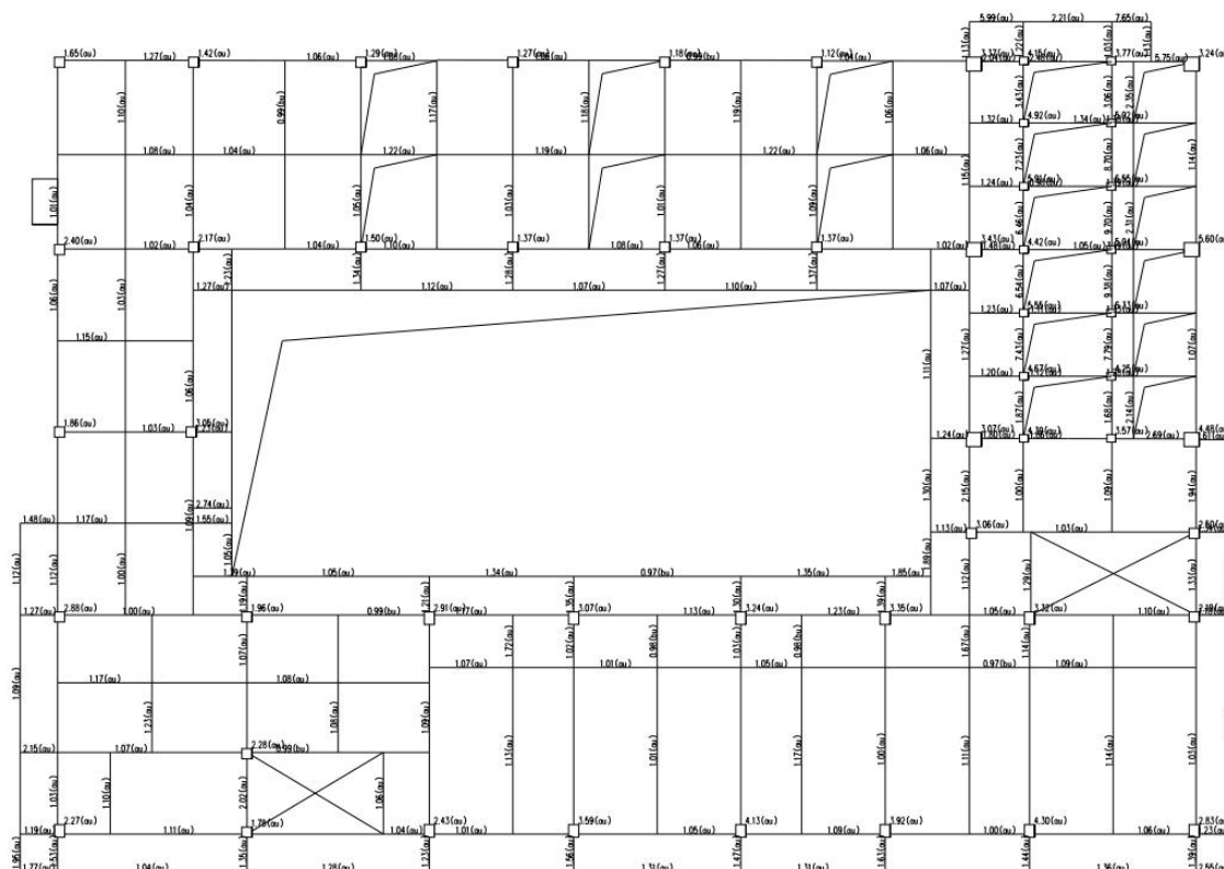
图 7.2.3 第 1 层砗抗力与效应比简图
