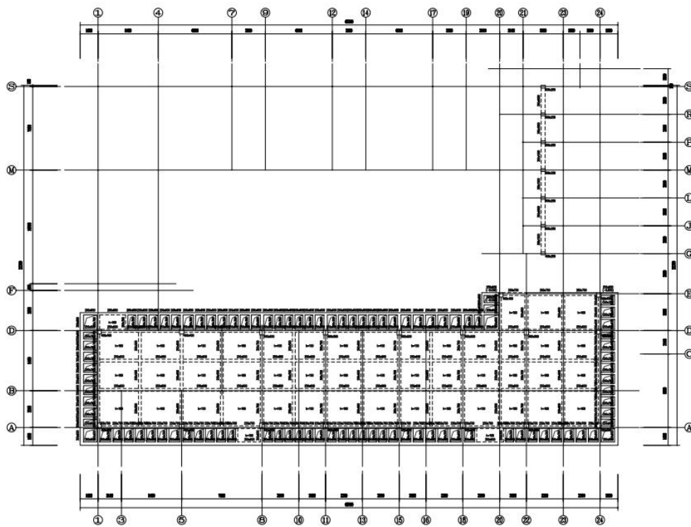
二层结构平面图
