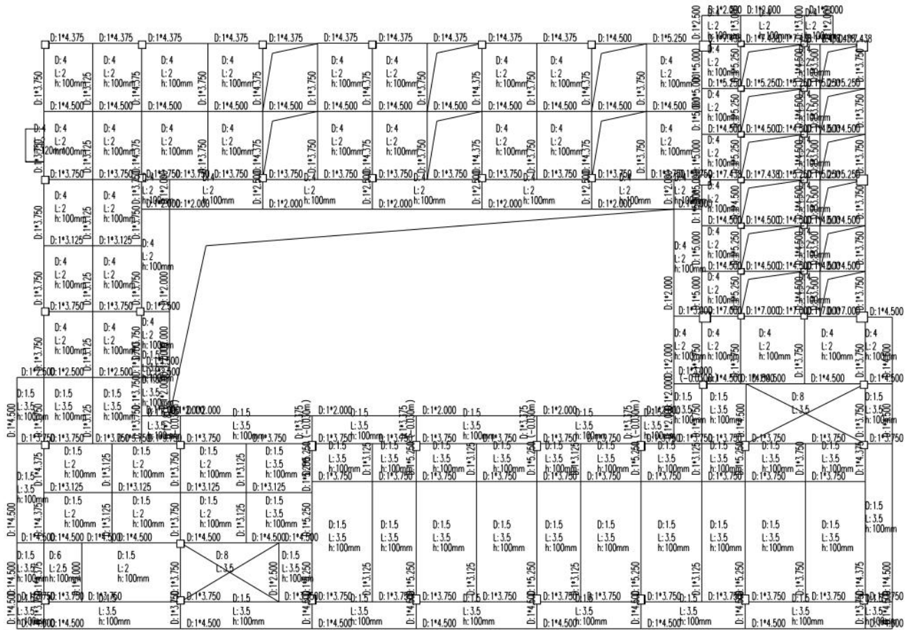
附图 3: 平面荷载图
