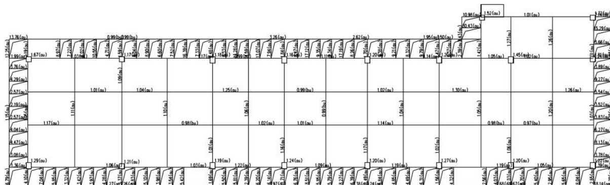
图 7.2.4 第 2 层砗抗力与效应比简图
