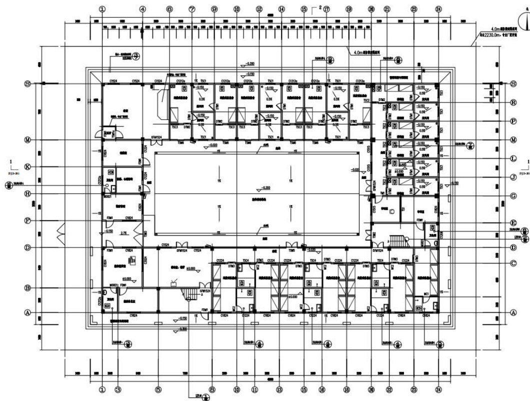
一层平面图
