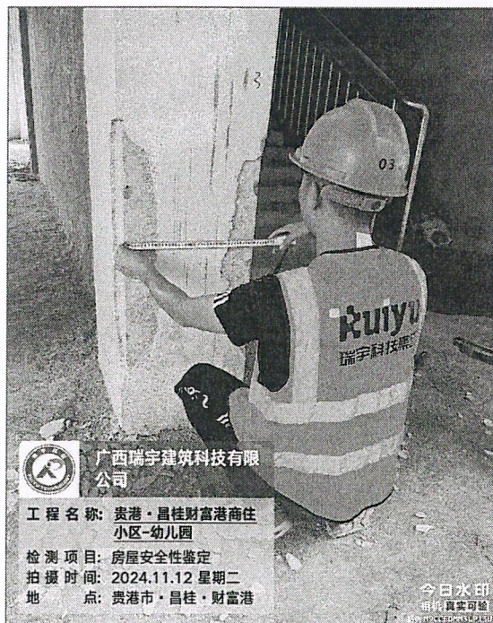
截面尺寸测量
