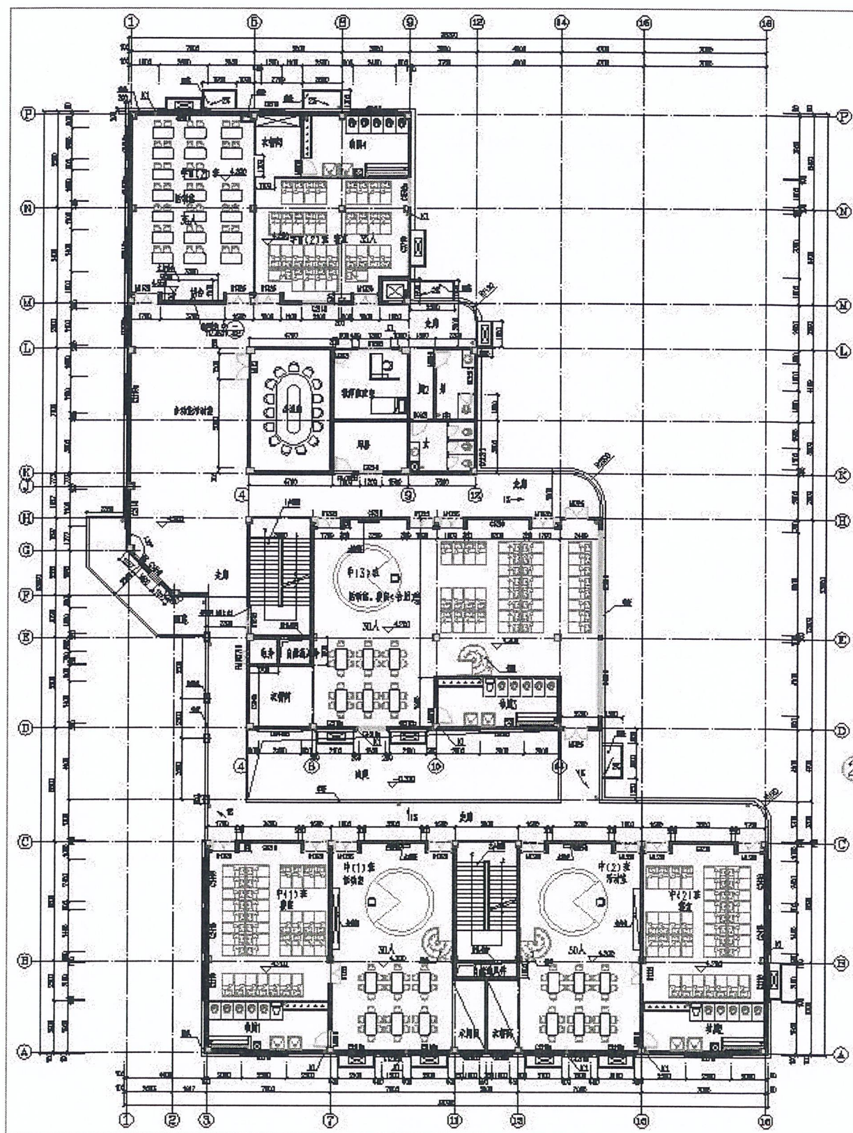
二层平面图
