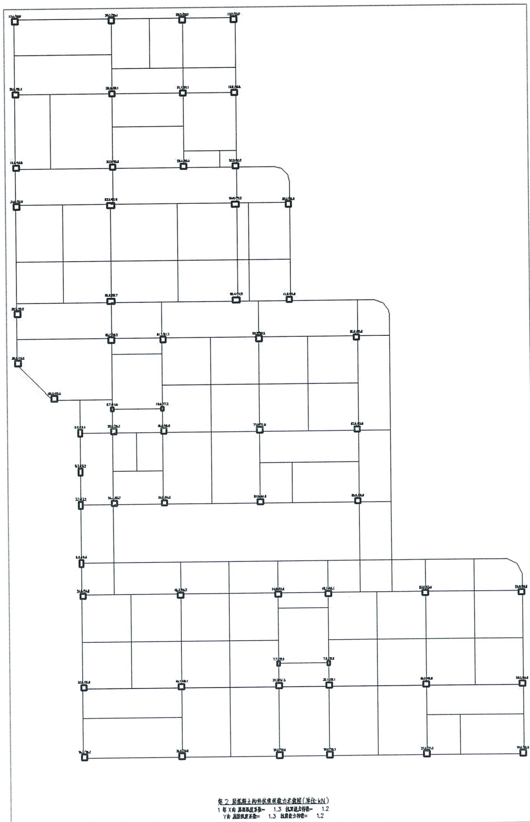
图 9.5.2 2 层混凝土柱梁抗震承载力验算结果
