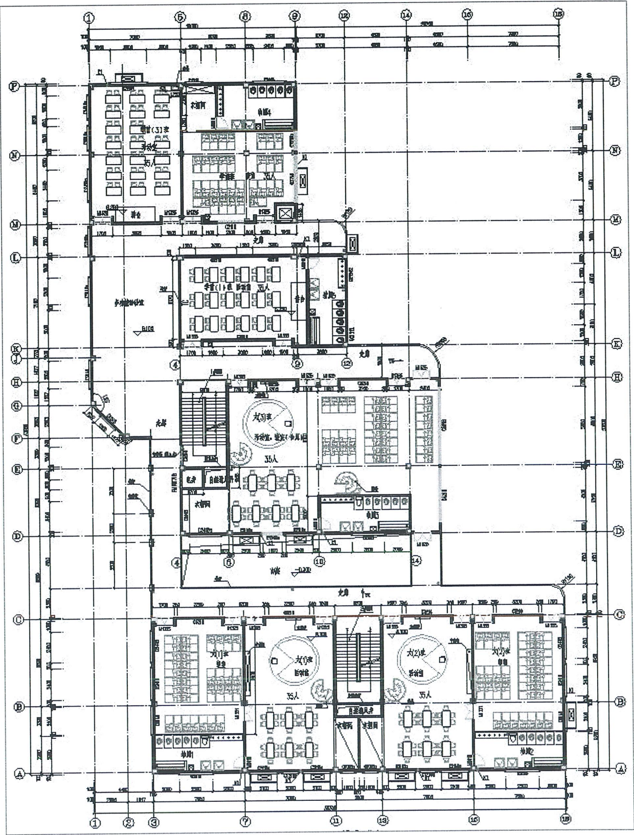
三层平面图
