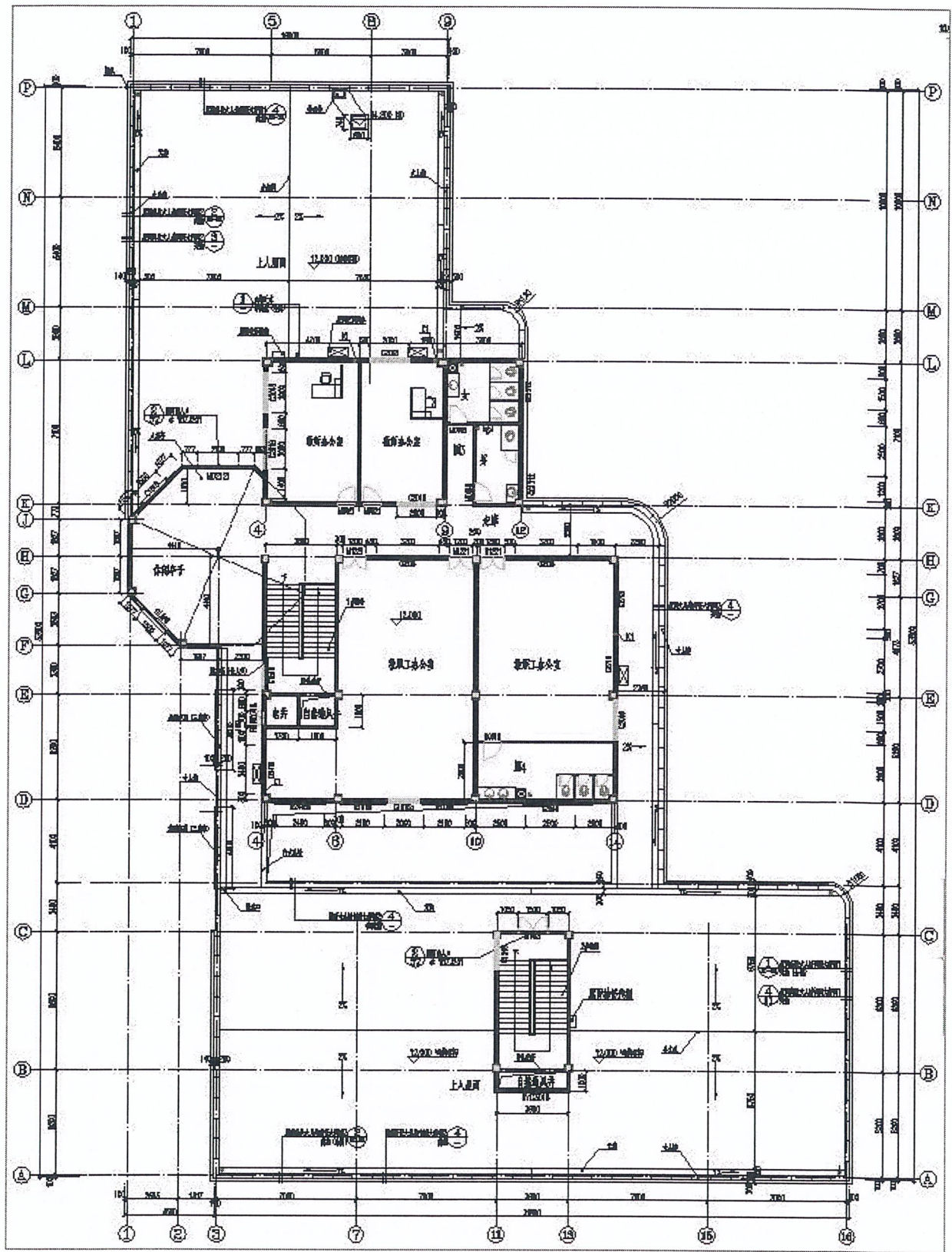
四层平面图
