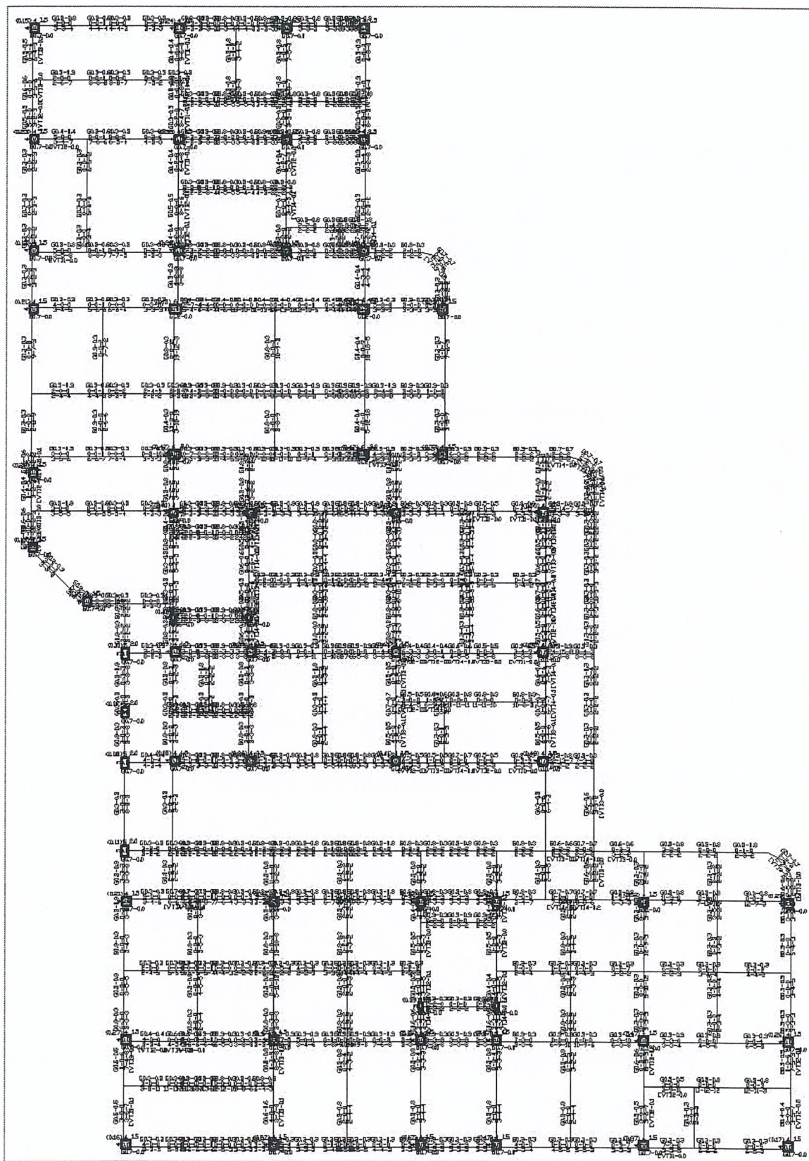
图 7.2.1 第 1 层砼构件配筋验算应力简图
