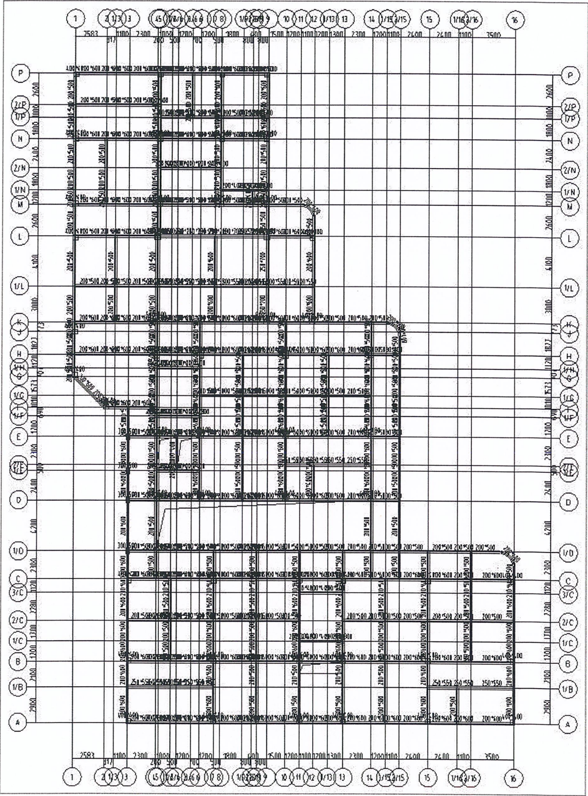
一层结构平面图
