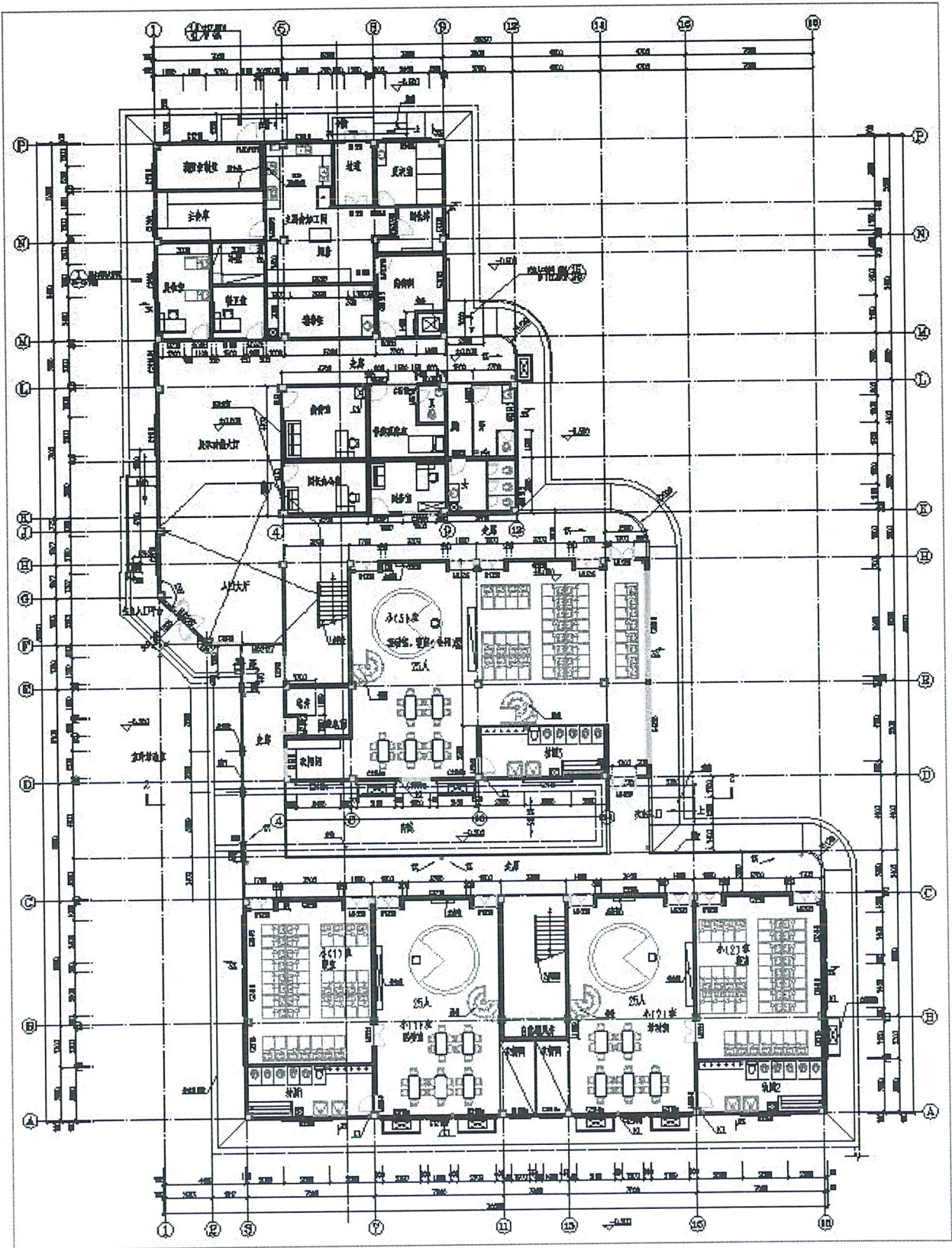
一层平面图
