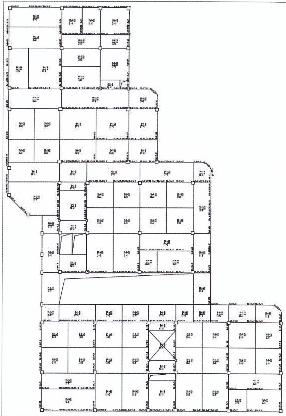
一层平面荷载图
