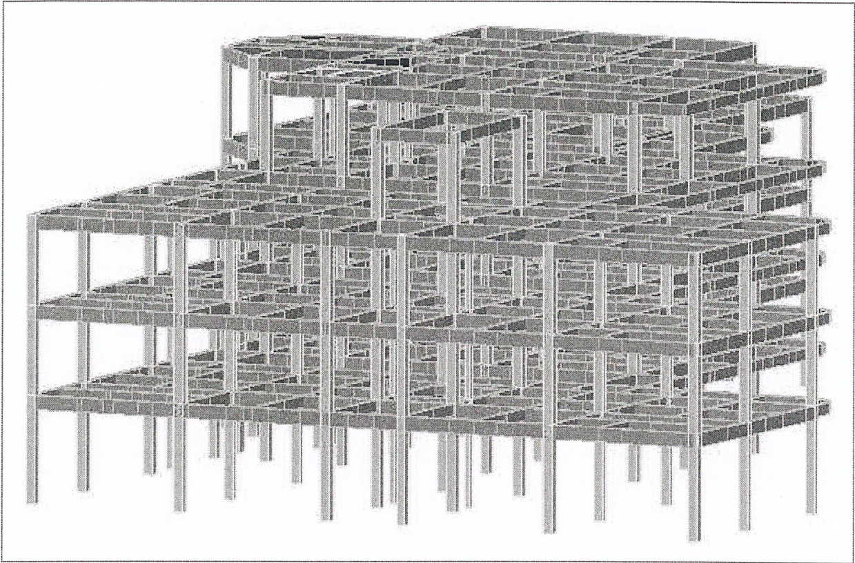
图7.1 结构模型简图
