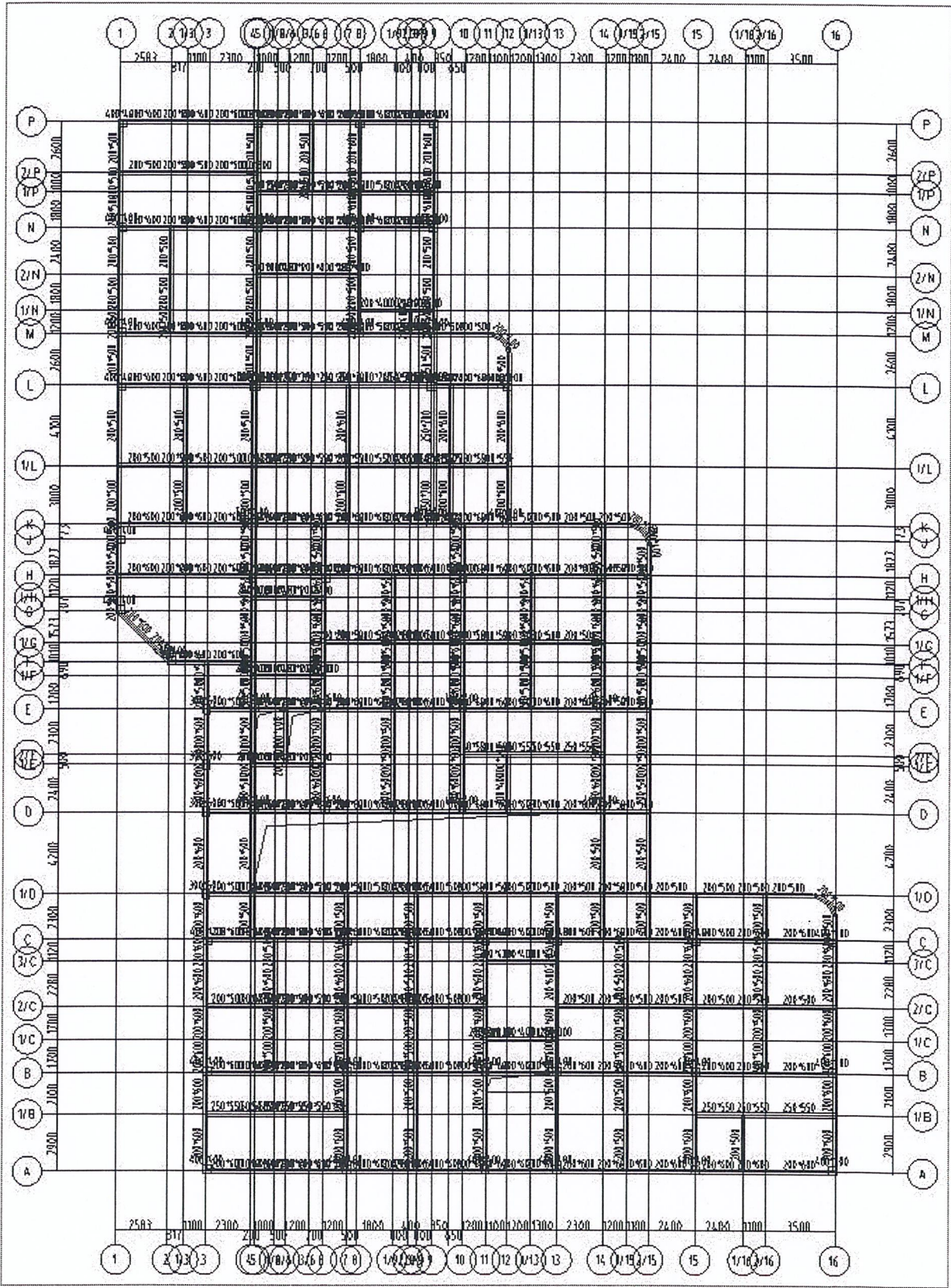
三层结构平面图
